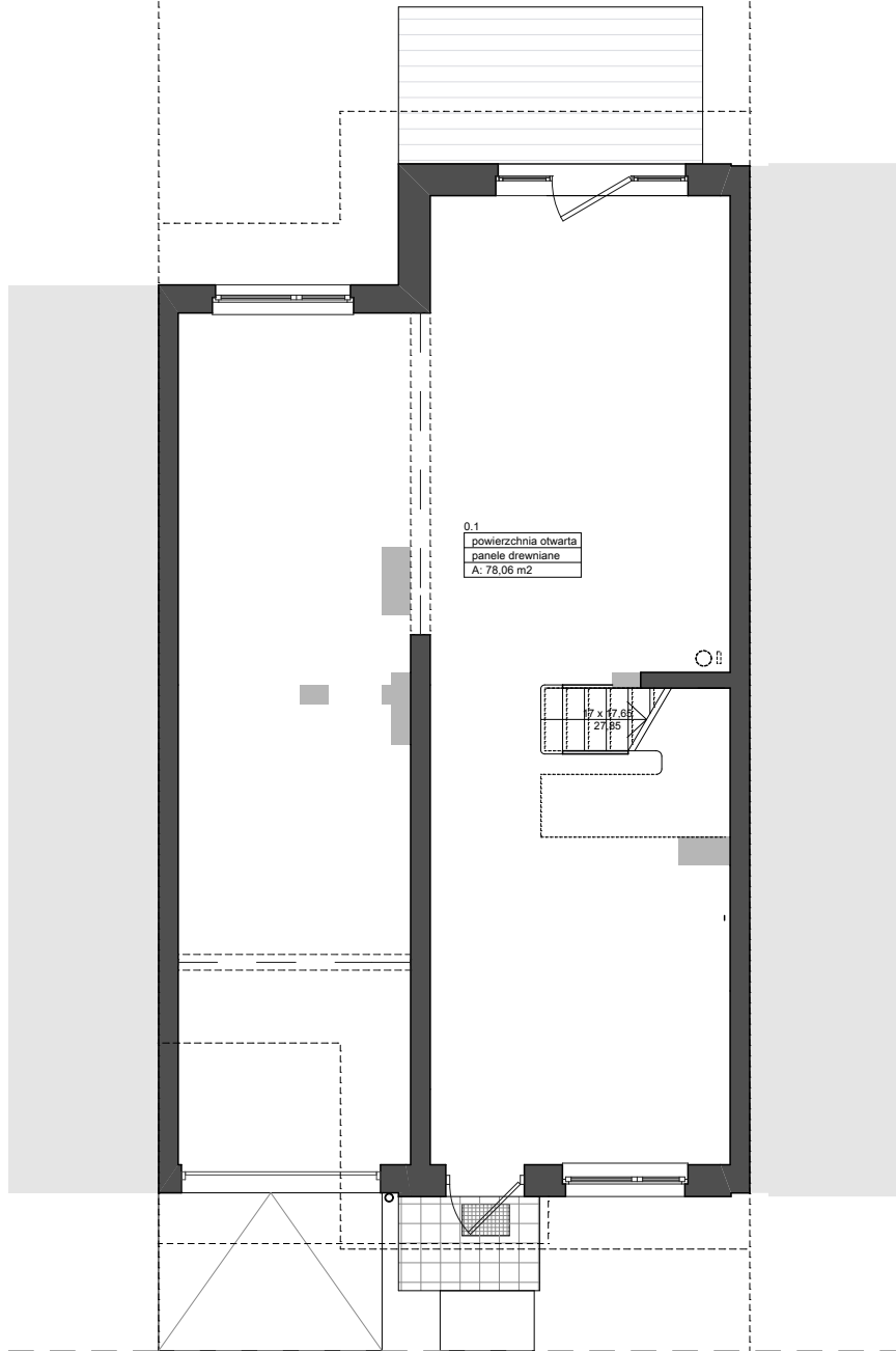
RZUT PARTERU
