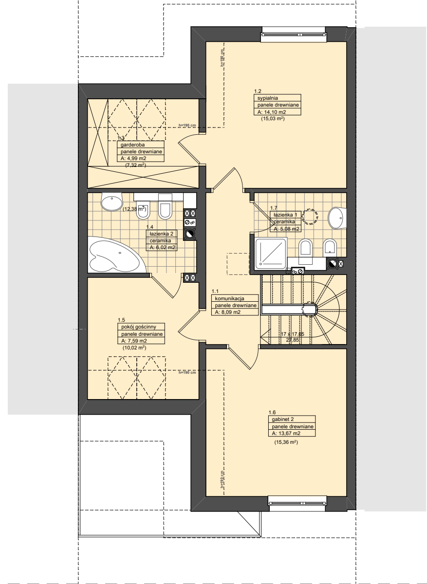
RZUT PIĘTRA
