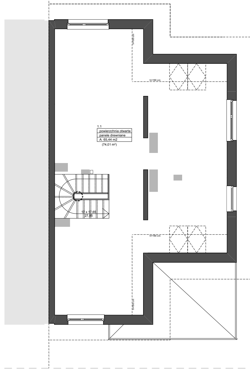
RZUT PIĘTRA
