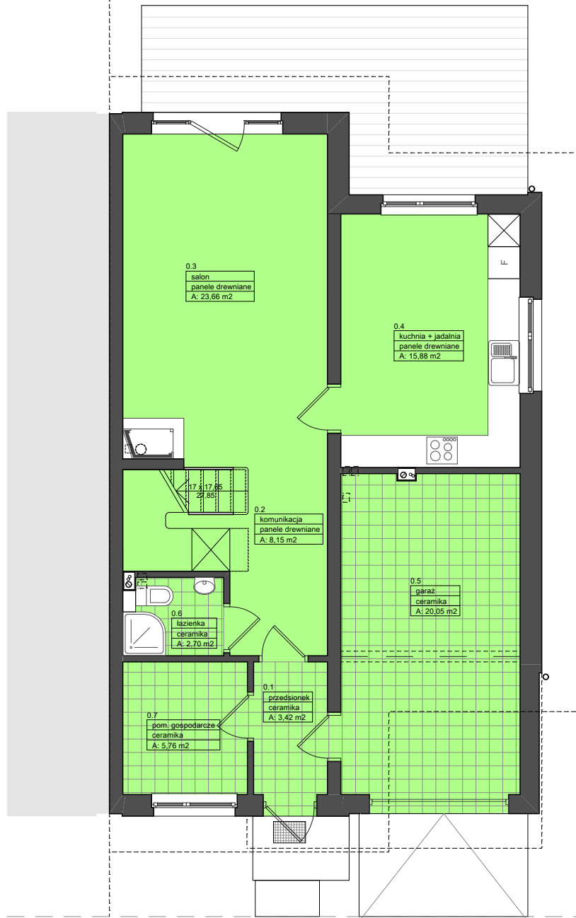
RZUT PARTERU
