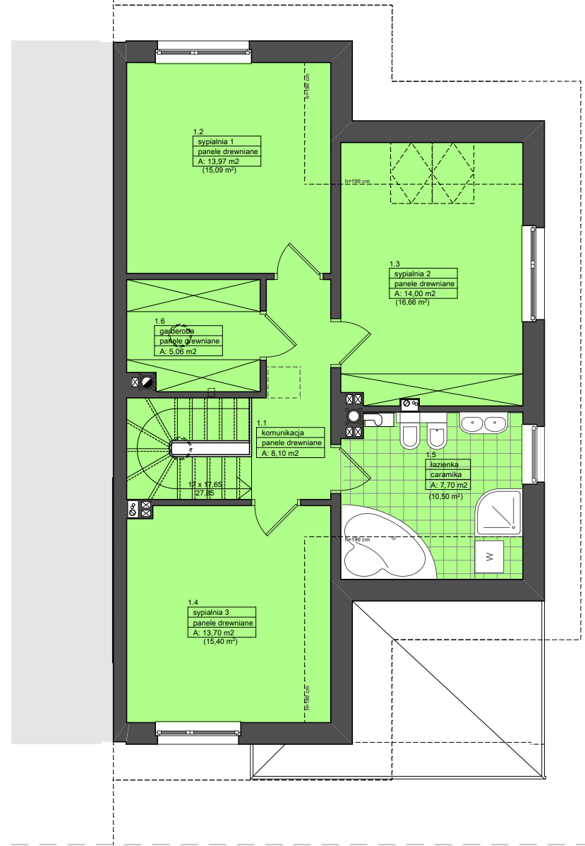
RZUT PIĘTRA
