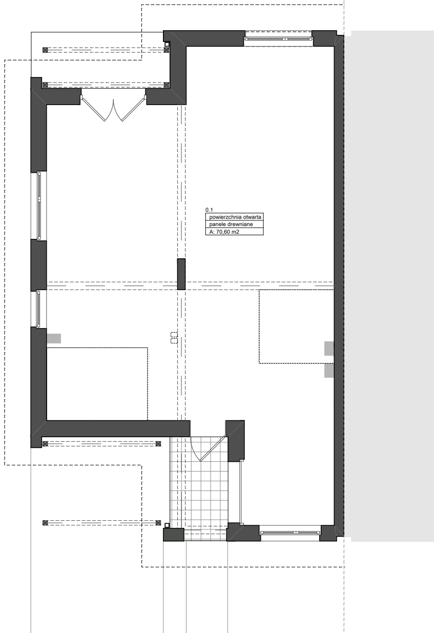
RZUT PARTERU
