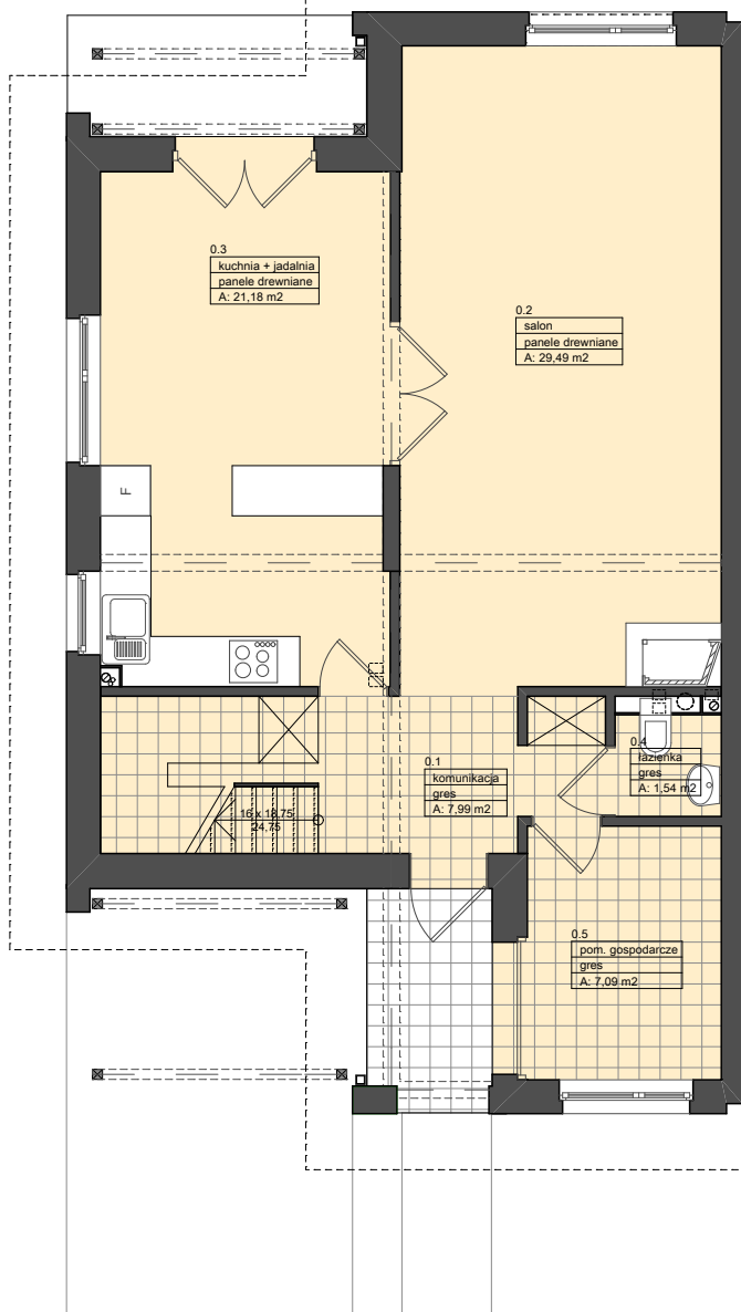
RZUT PARTERU
