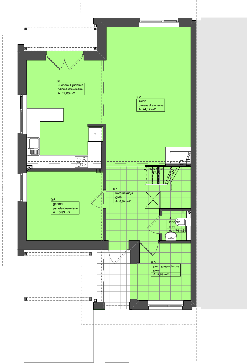
RZUT PARTERU
