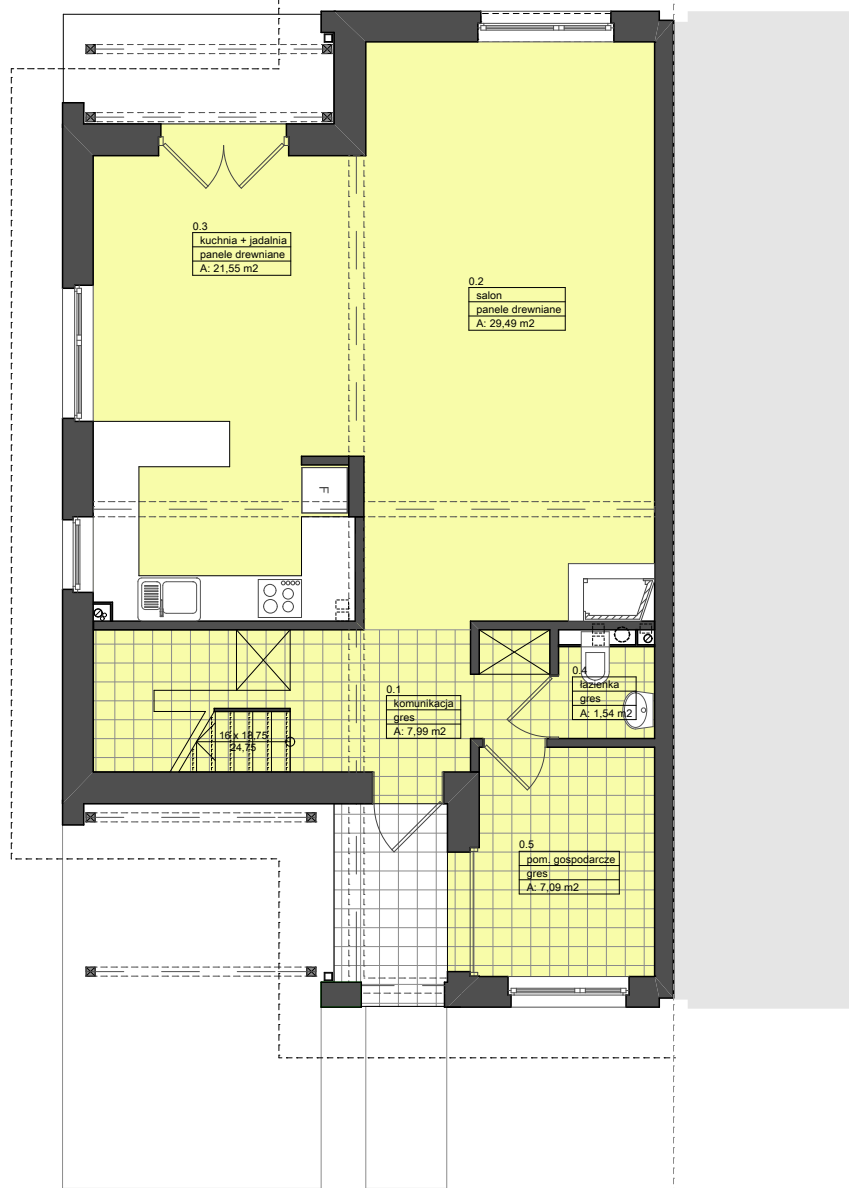
RZUT PARTERU
