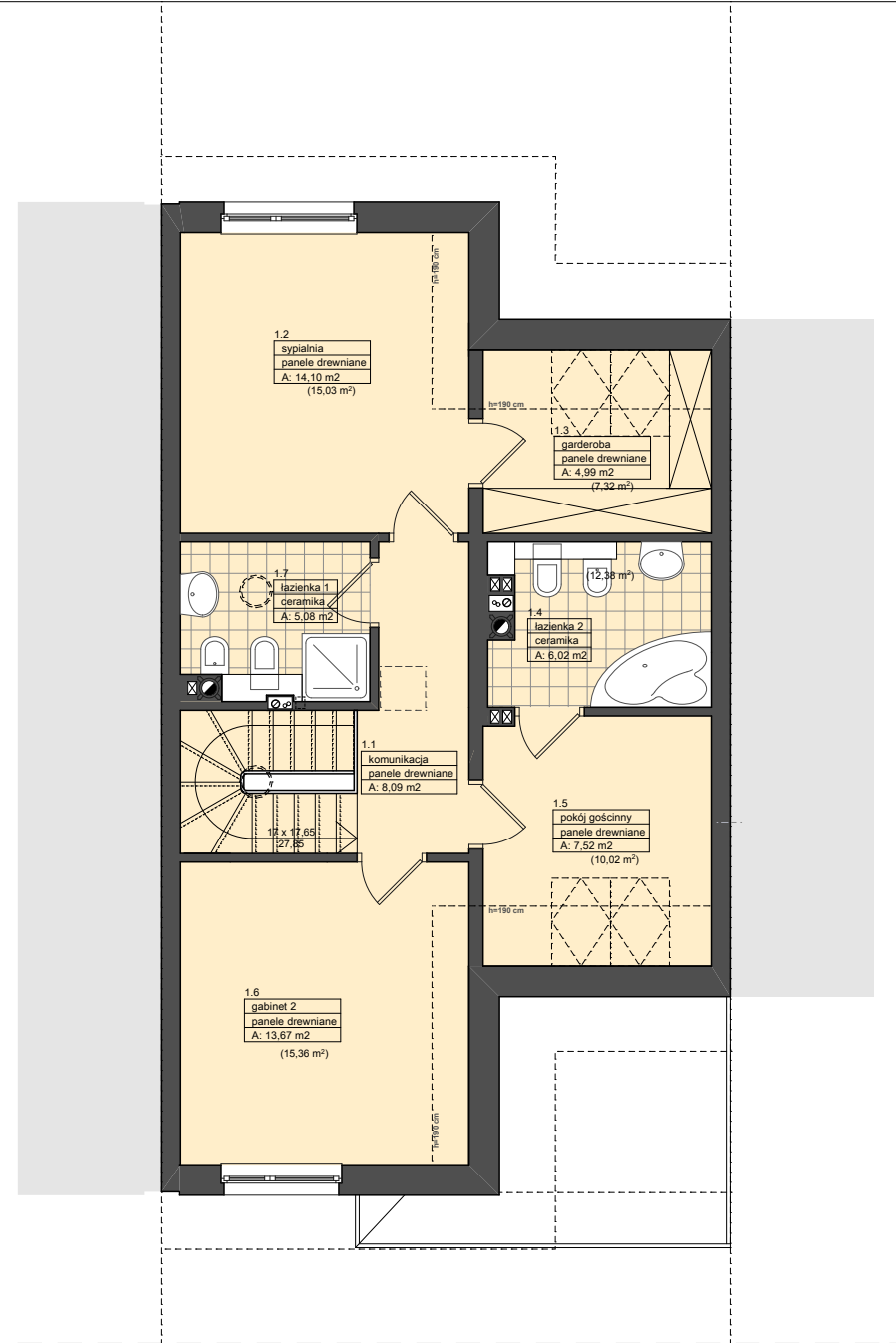
RZUT PIĘTRA
