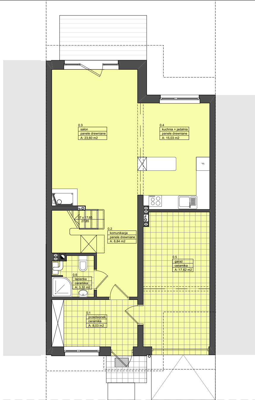
RZUT PARTERU
