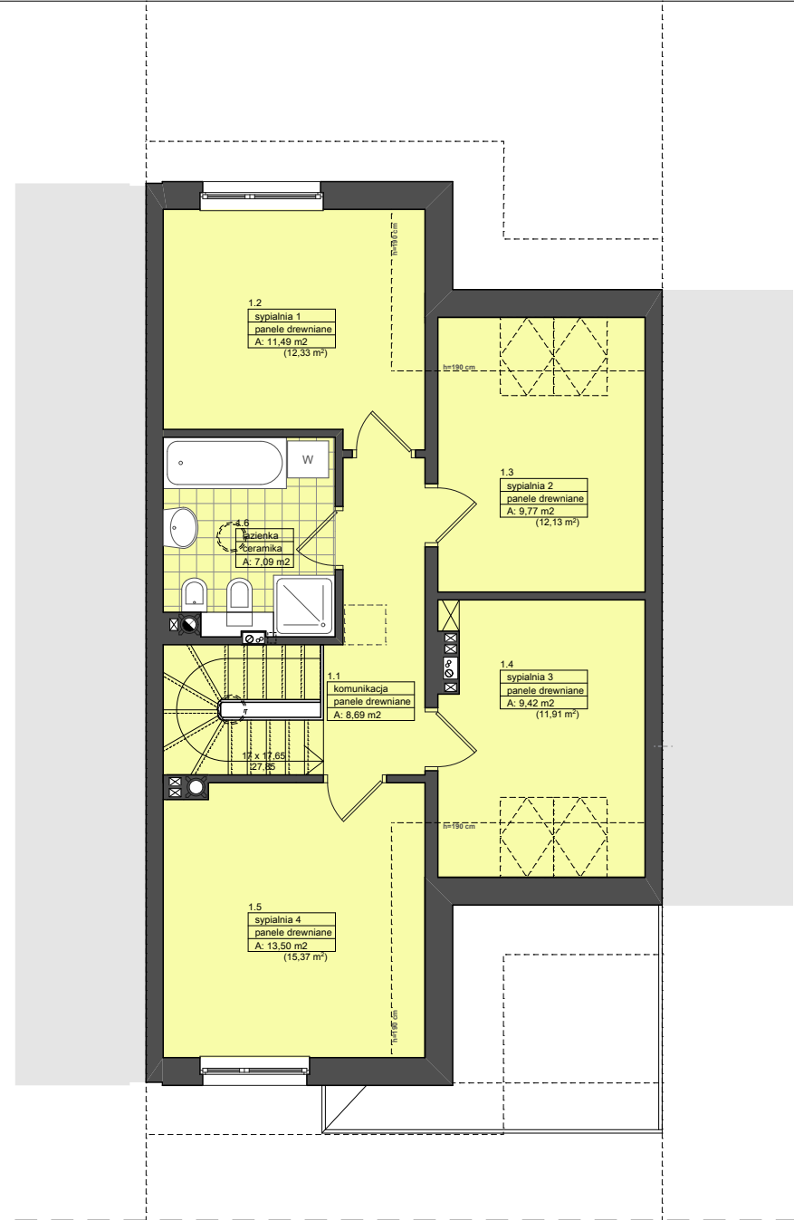
RZUT PIĘTRA
