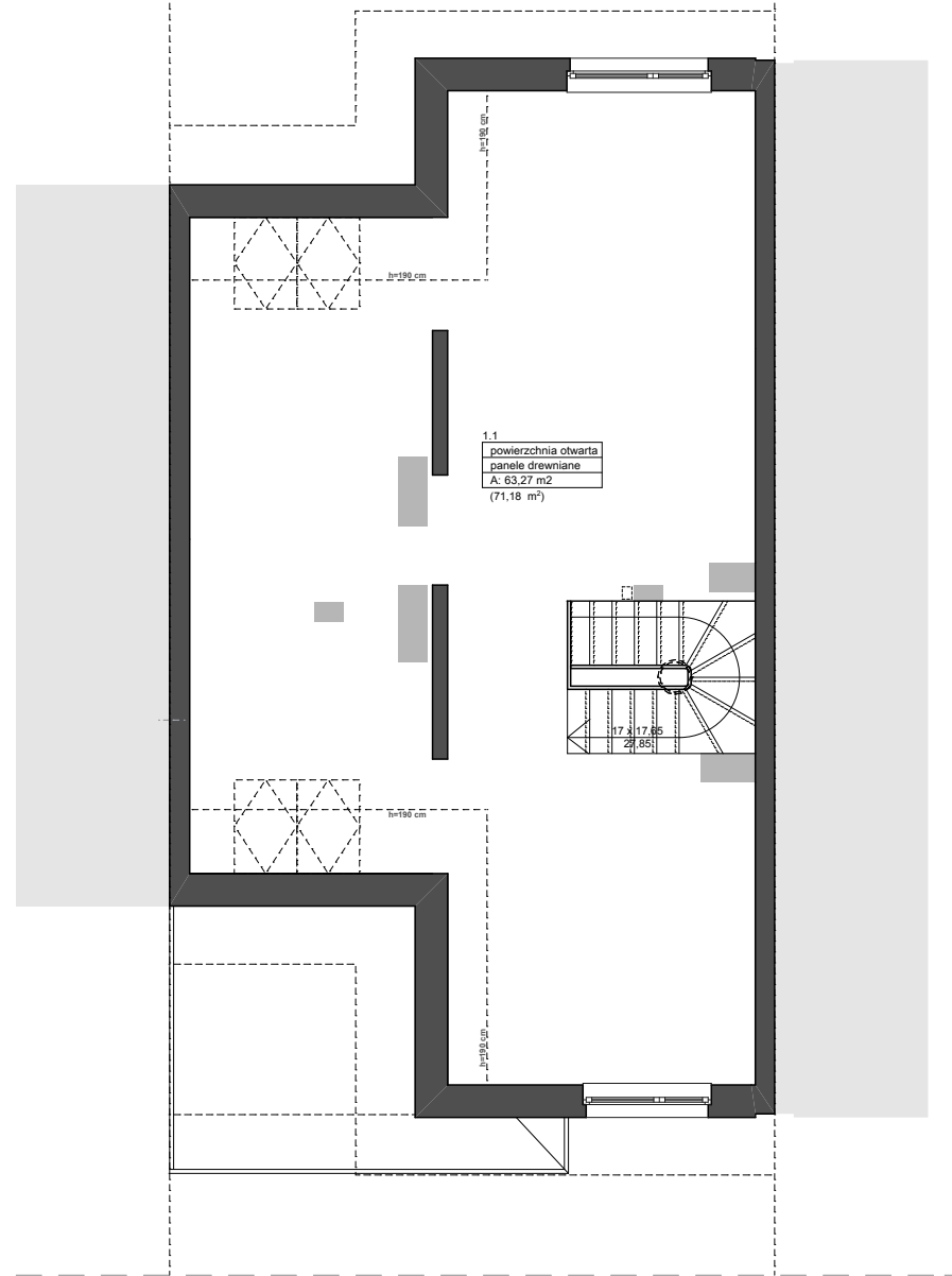
RZUT PIĘTRA
