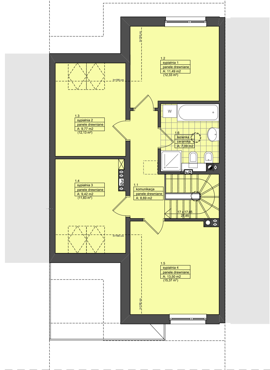
RZUT PIĘTRA
