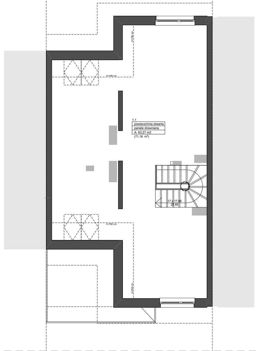
RZUT PIĘTRA
