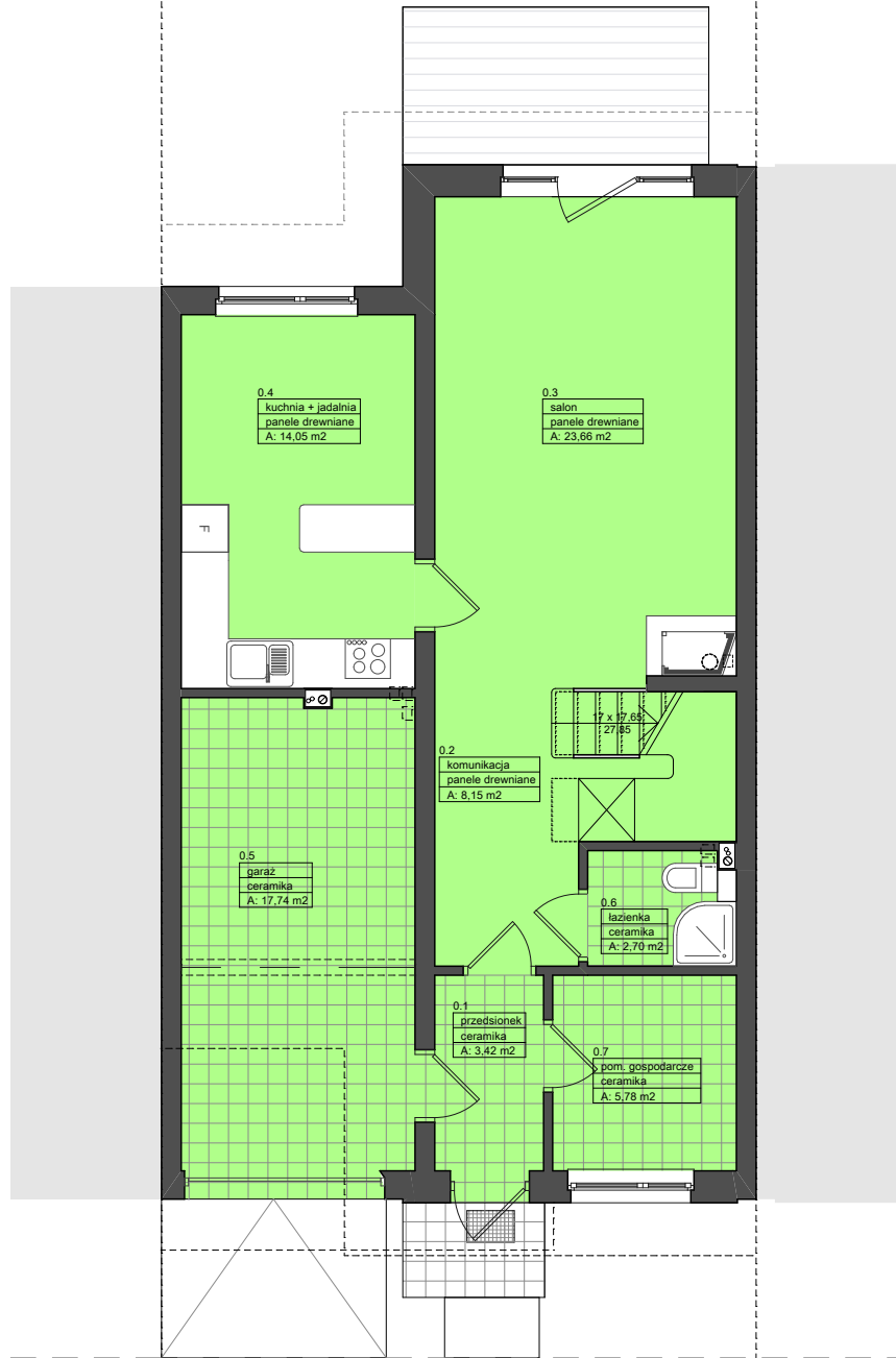
RZUT PARTERU
