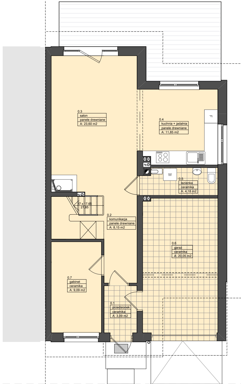
RZUT PARTERU
