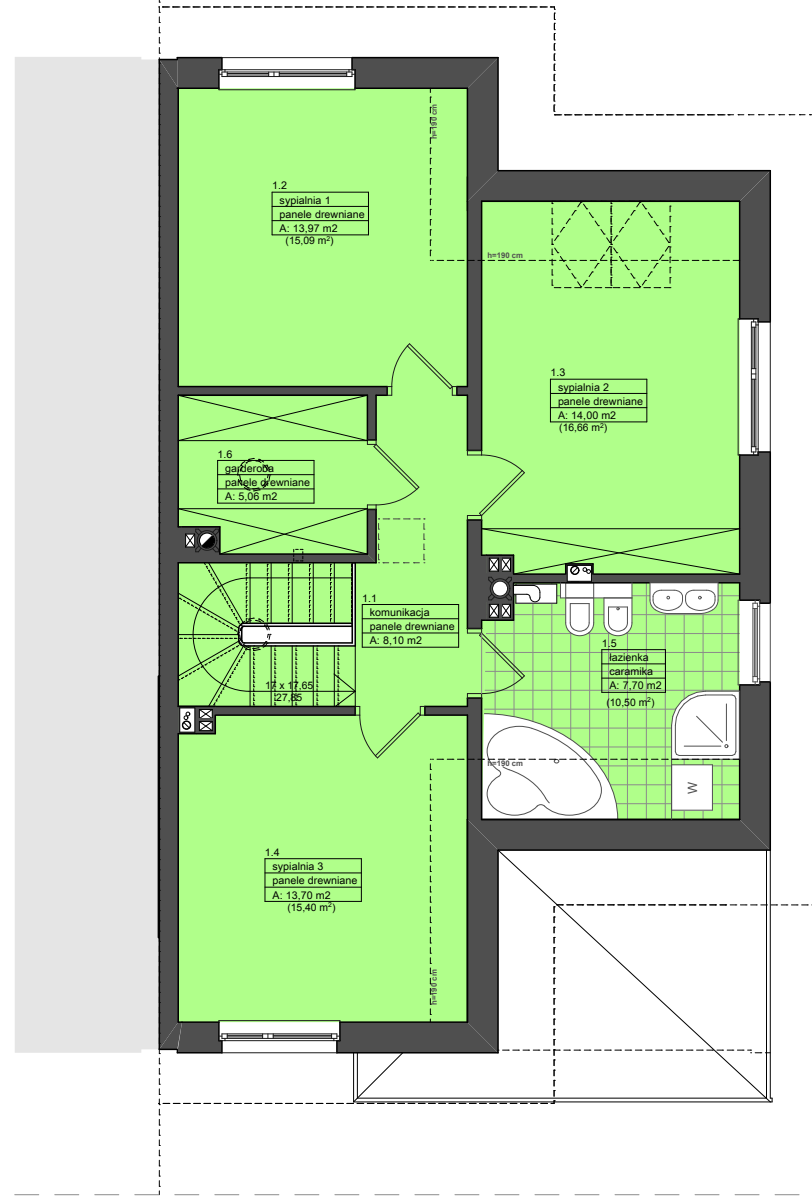
RZUT PIĘTRA
