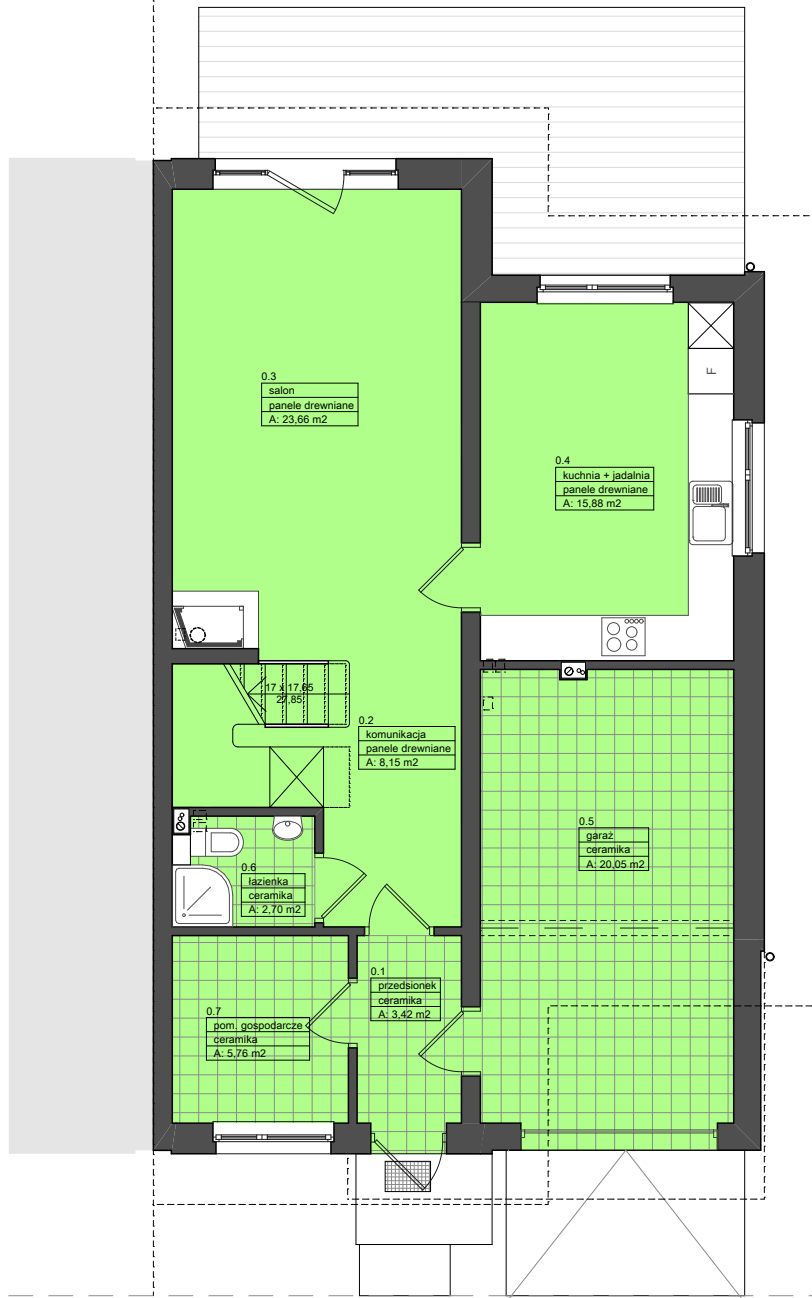
RZUT PARTERU
